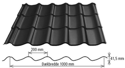
Teglstenprofil
